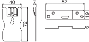
壁金具
