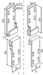
パネルにネジで金具を取り付け
