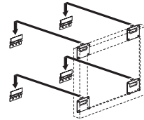
引掛け金具をセットした後に上部よりネジで固定します。
