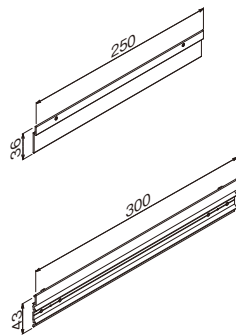
フレームにネジで金具を取り付け
